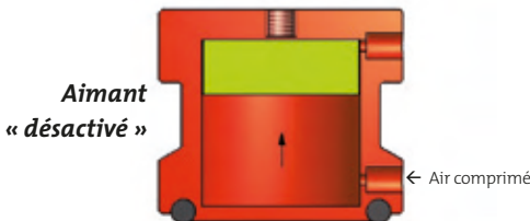
AIMANT VERS LE HAUT → DÉPOSE
