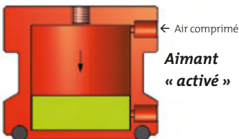
AIMANT VERS LE BAS → PRÉHENSION
